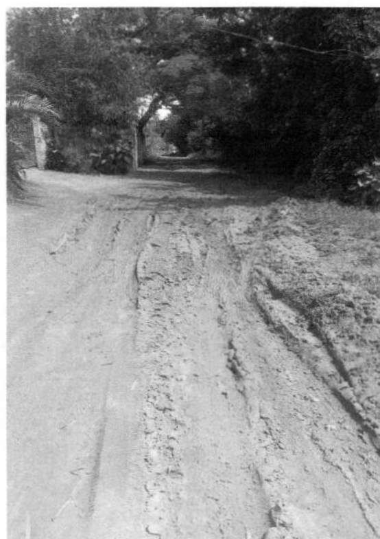
NIVELAMENTO E CASCALHAMENTO na Rua Ceará, Santo Ângelo - Mogi das Cruzes
